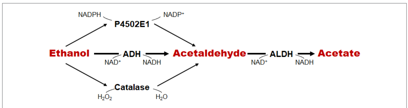
그림 1. 알코올 대사과정
